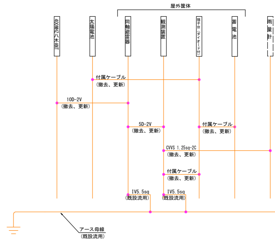
配線系統図
