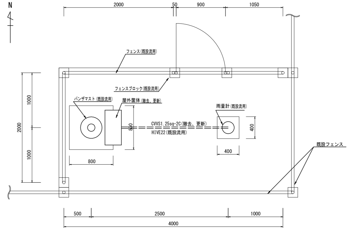
敷地平面図
