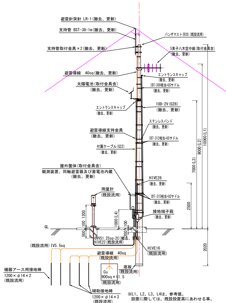
基本実装図(標準図)
